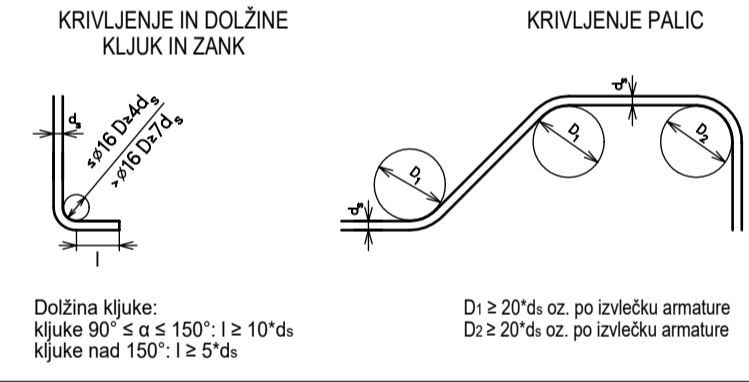
KRIVLJENJE ARMATURE PO SIST EN 1992-1-1
