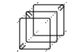
POLAGANJE STREMEN odprtine stremen zamkali
